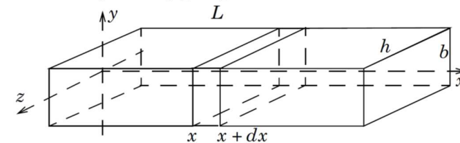
Figure 1 - Vibrations longitudinales d'une lame parallélépipédique
